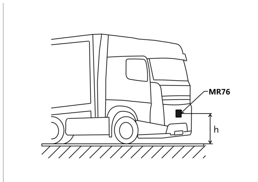
图 3 MR76 雷达垂直安装示意图
