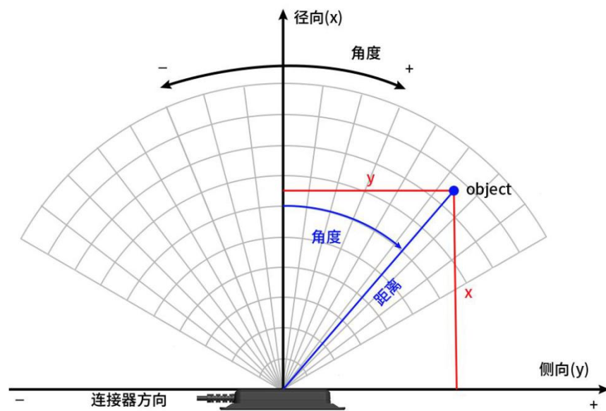
图 5 雷达方向说明示意图
