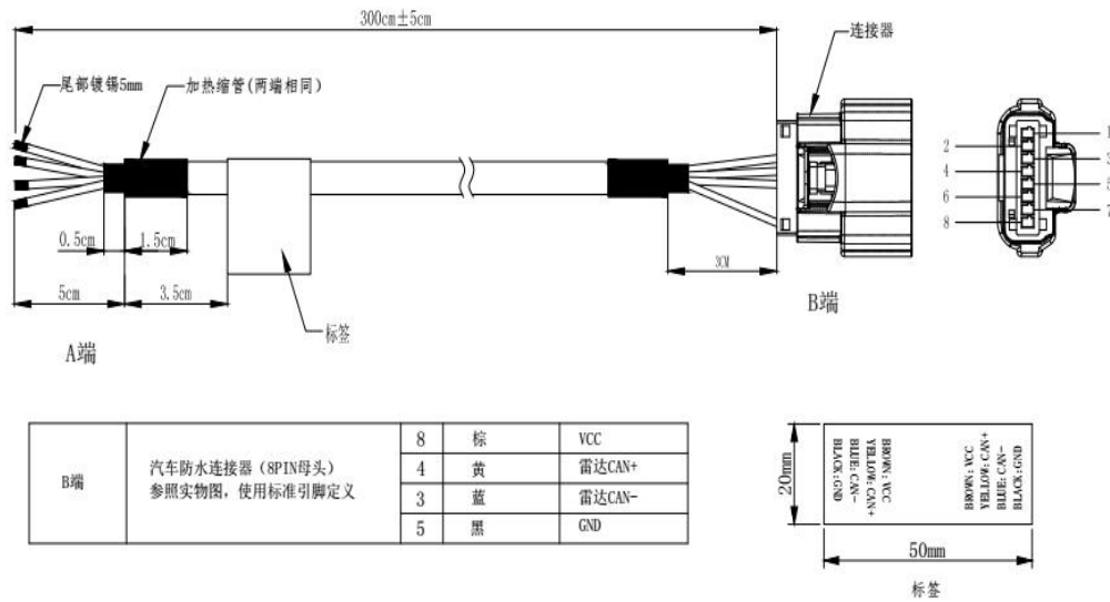
图 10 CAN 接口线束连接示意图
