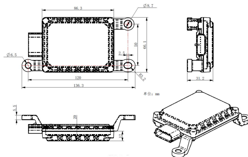
图 12 MR76 带壳尺寸图
