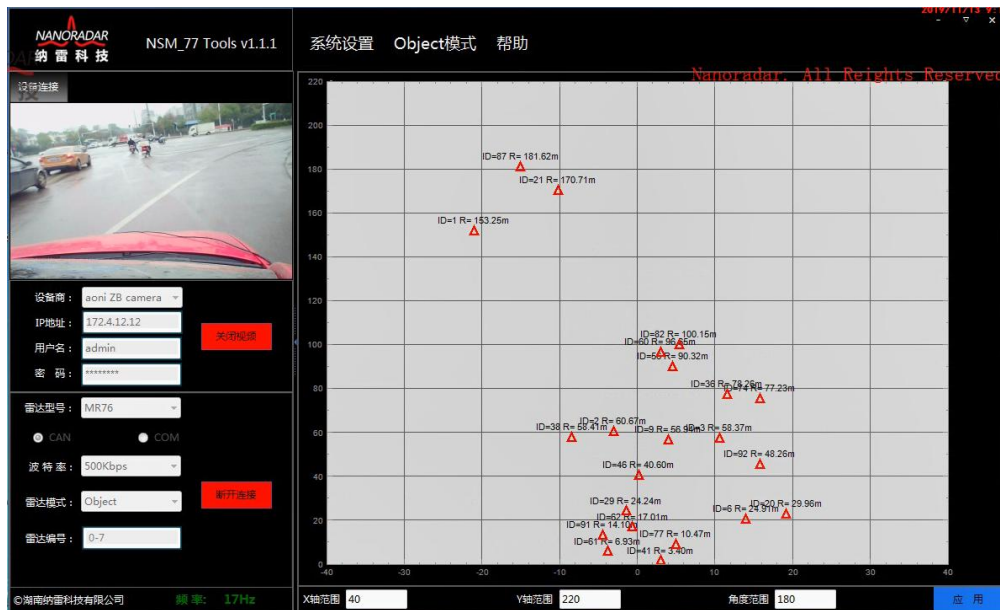
图 9 雷达上位机测试界面
