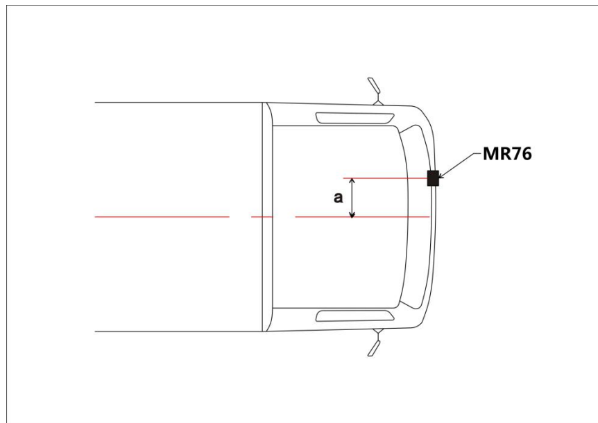
图 4 MR76 雷达水平安装示意图
